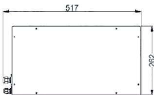
Vnitřní jednotka čelní pohled:
